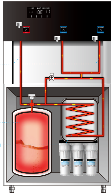
隔夜水智能排放示意圖： 管道及龍頭智能消毒示意圖：
