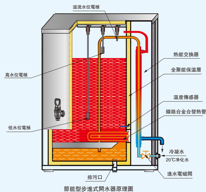
節能型步進式開水器原理圖
