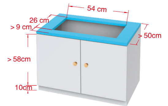
安裝開孔圖
