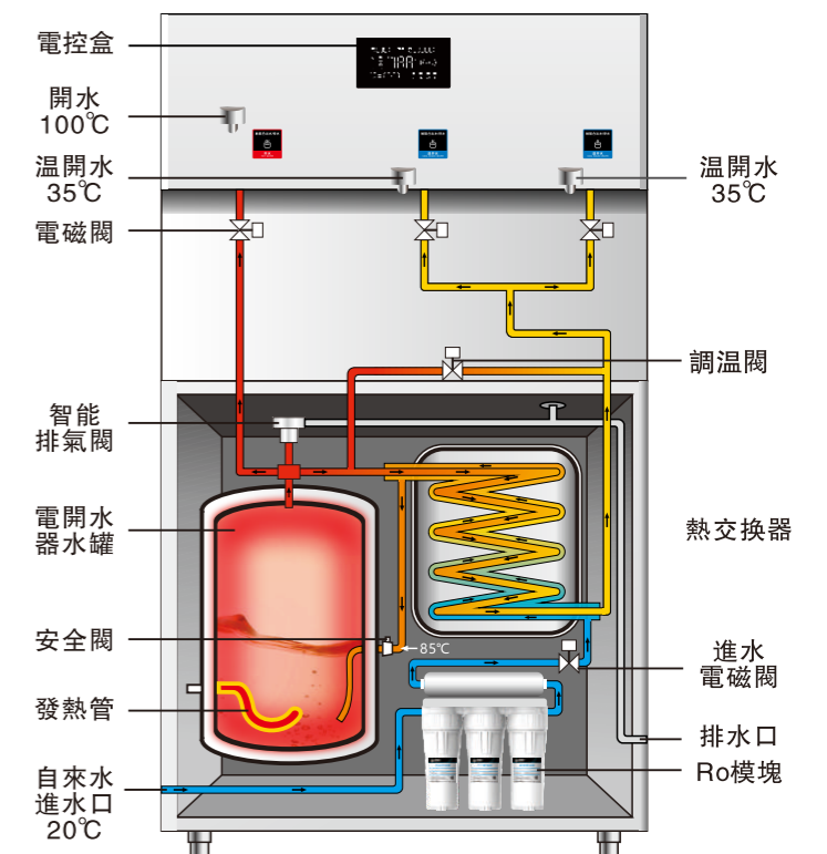
圖2 碧麗常壓式節能飲水機專利原理圖
