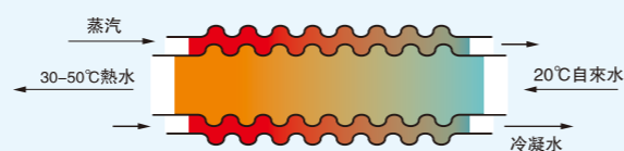
蒸汽回收裝置原理圖
