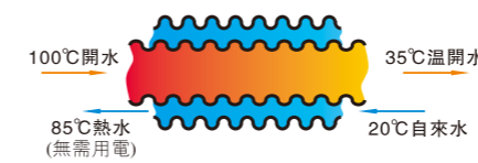
圖2 第三代熱交換器節能原理圖
